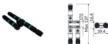
Micro derivatore 3 vie 2M+1F 10A 2 poli 0,25-1,5mm 2 (23-16AWG) Øcavo 5,8-6,9mm (0,23-0,27") - IP68
