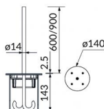
Plaque de base avec boulons d'ancrage
